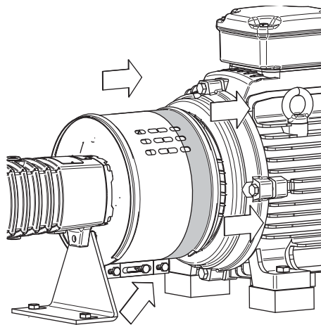
Figura 12: Ajuste de la cubierta en la parte del motor.
