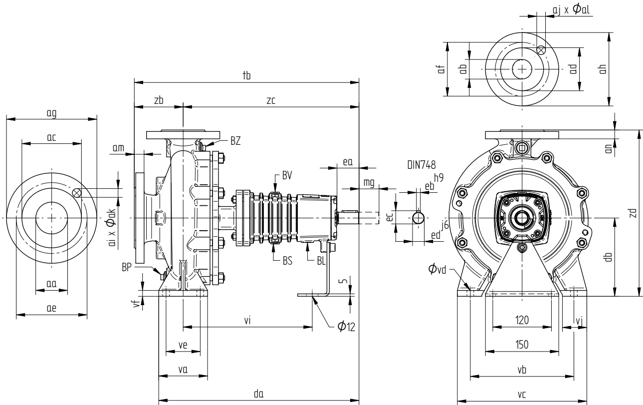
Figura 17: Dimensiones de la bomba.
