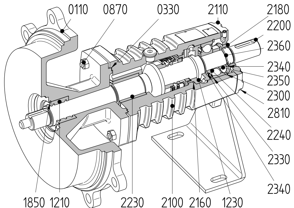
Figura 15: Cojinete L1 y junta mecánica de estanqueidad M1, M5).
