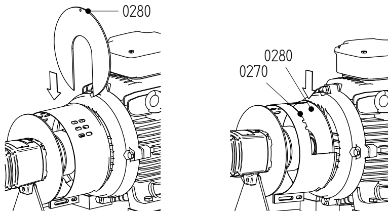
Figura 9: Instalación de la placa de montaje en la parte del motor.
