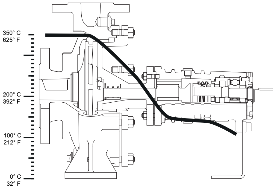
Figura 24: Disipación de temperatura en la bomba.
