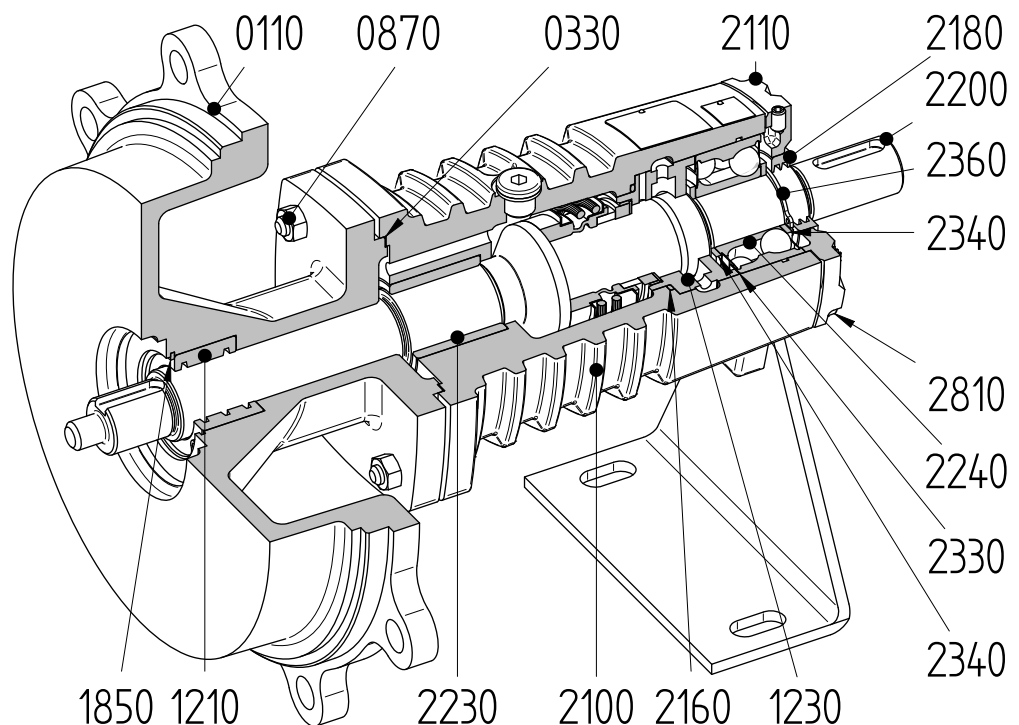
Figura 16: Cojinete L2 y junta mecánica de estanqueidad M1, M5).
